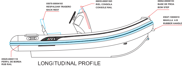
LONGITUDINAL PROFILE
