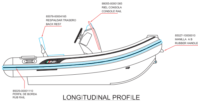
LONGITUDINAL PROFILE
